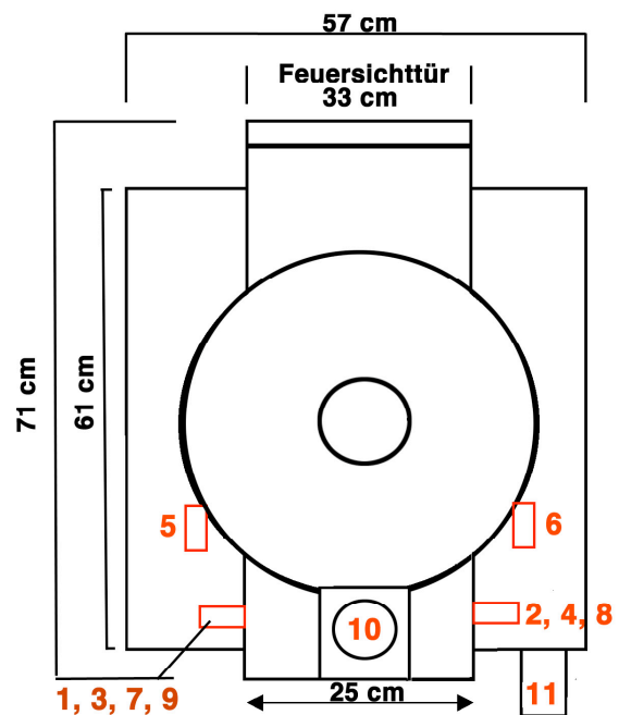
Sicht von oben (Skizze)
